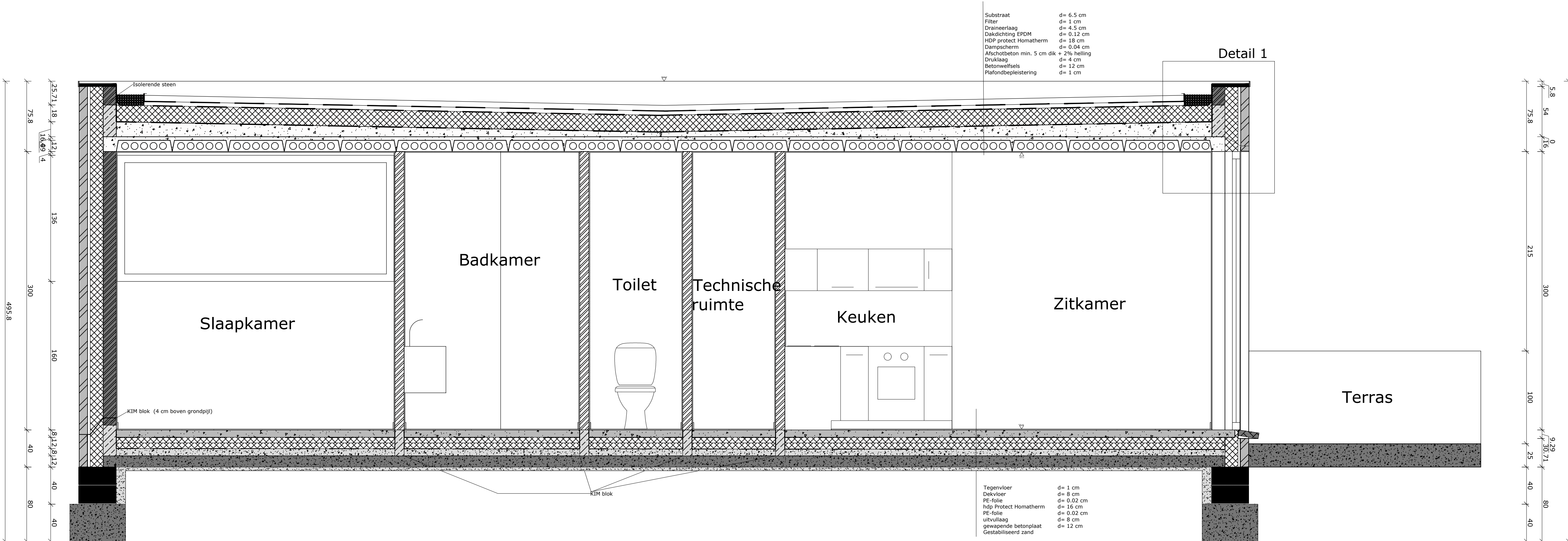
Snede AA' Schaal: 1/25
