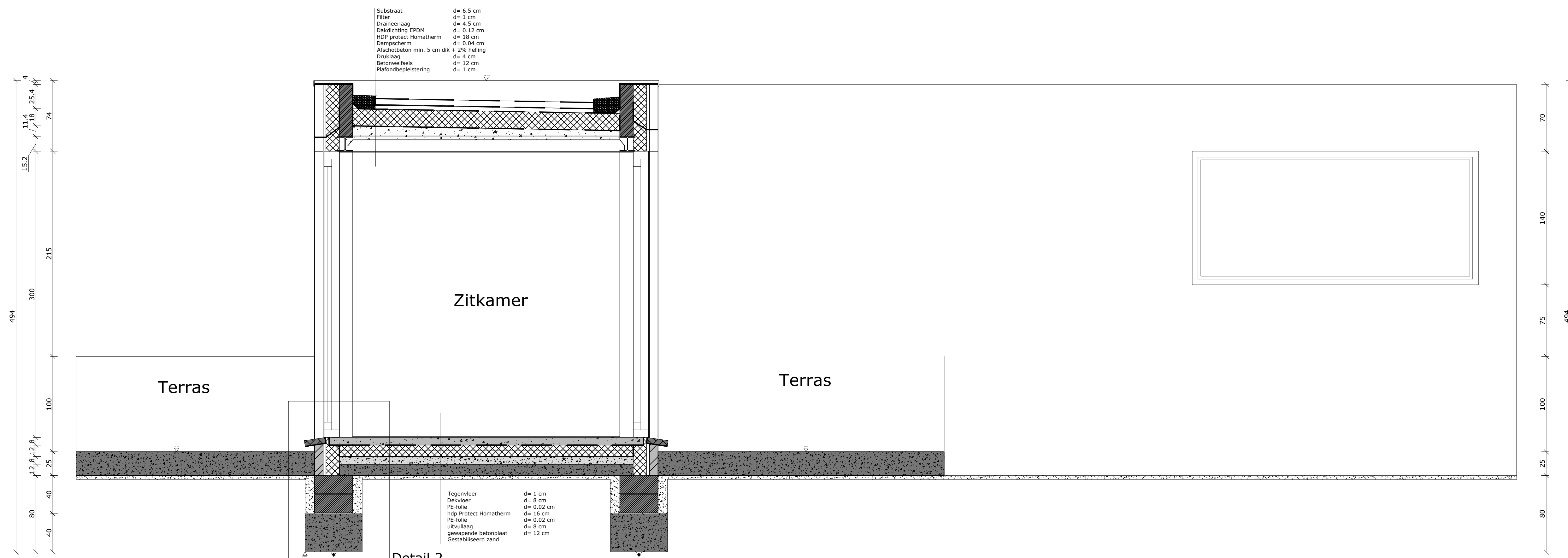
Snede BB' Schaal: 1/25
