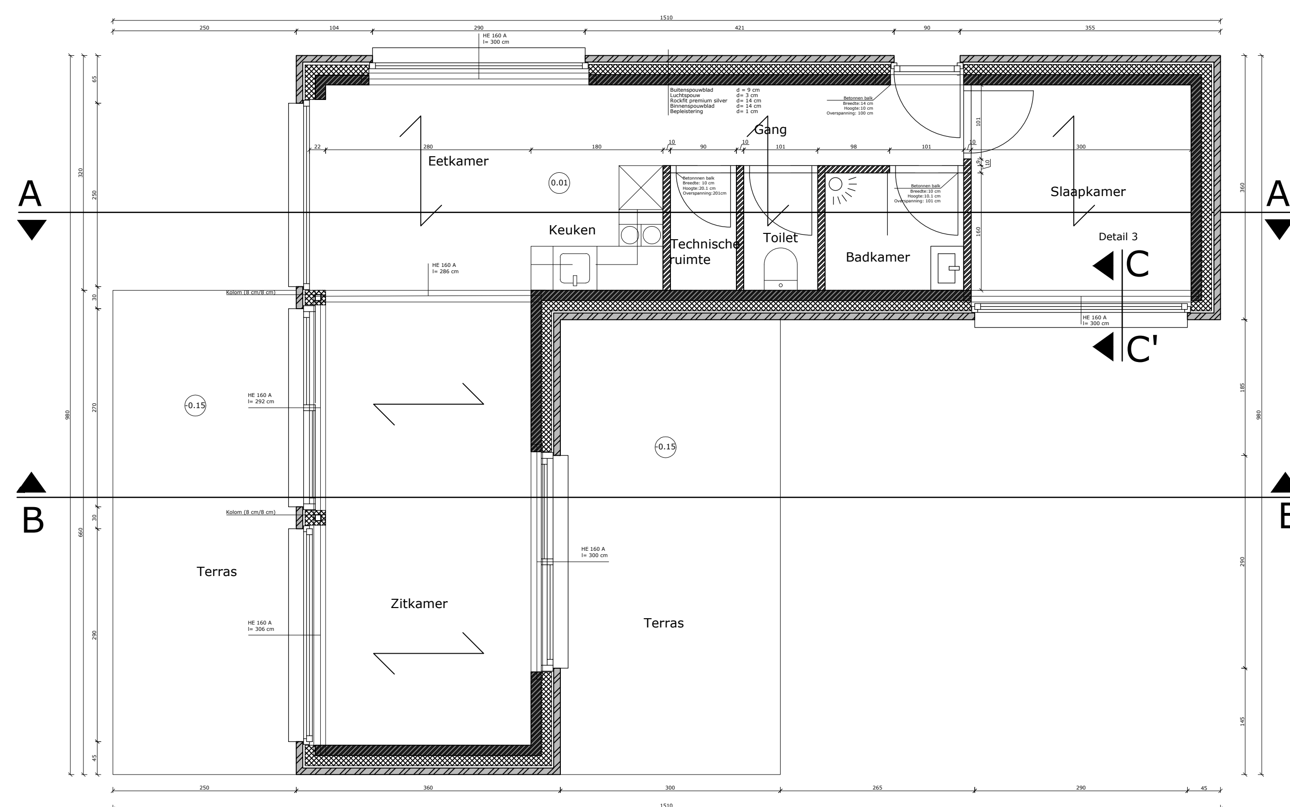
Grondplan
