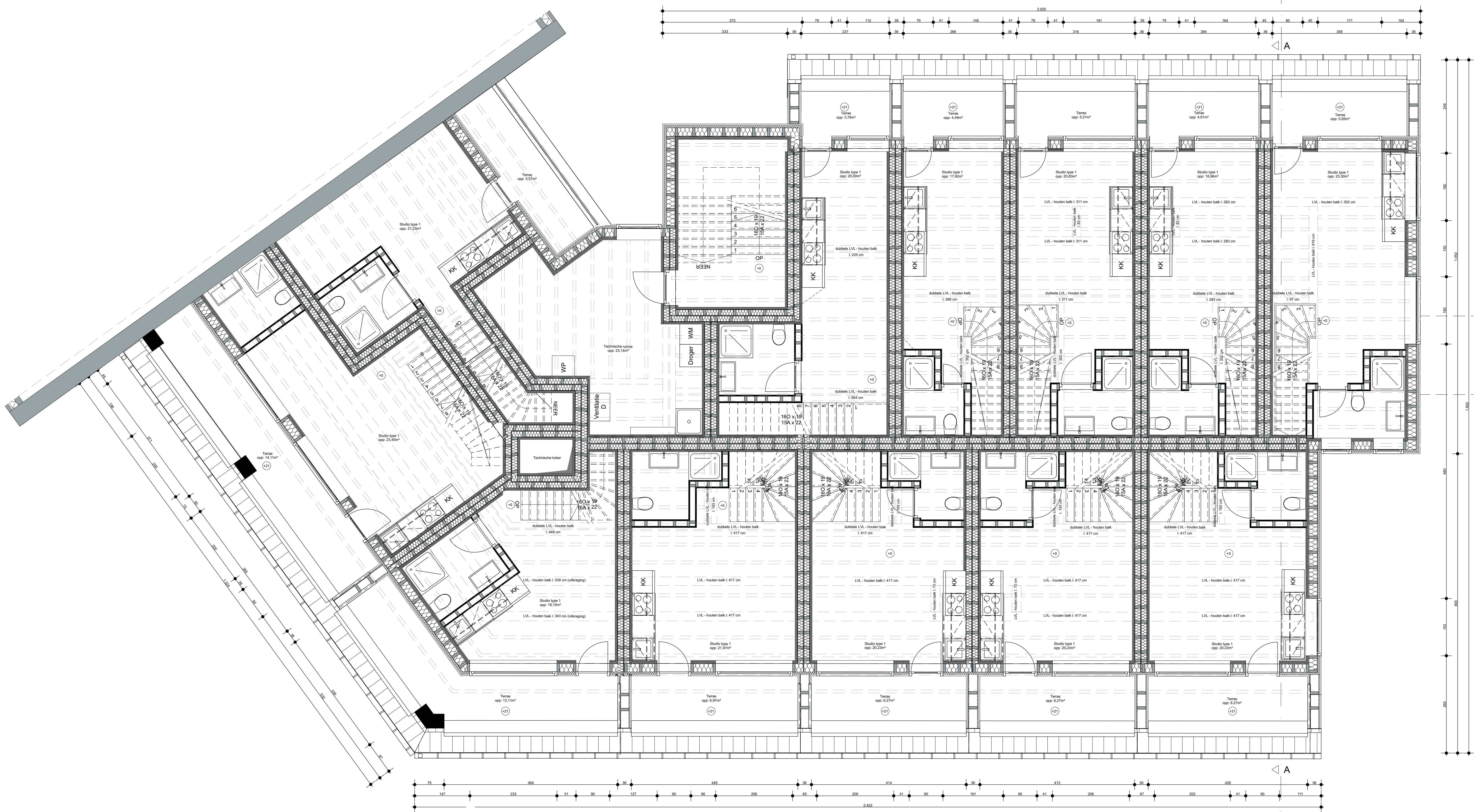
Grondplan gelijkvloers
