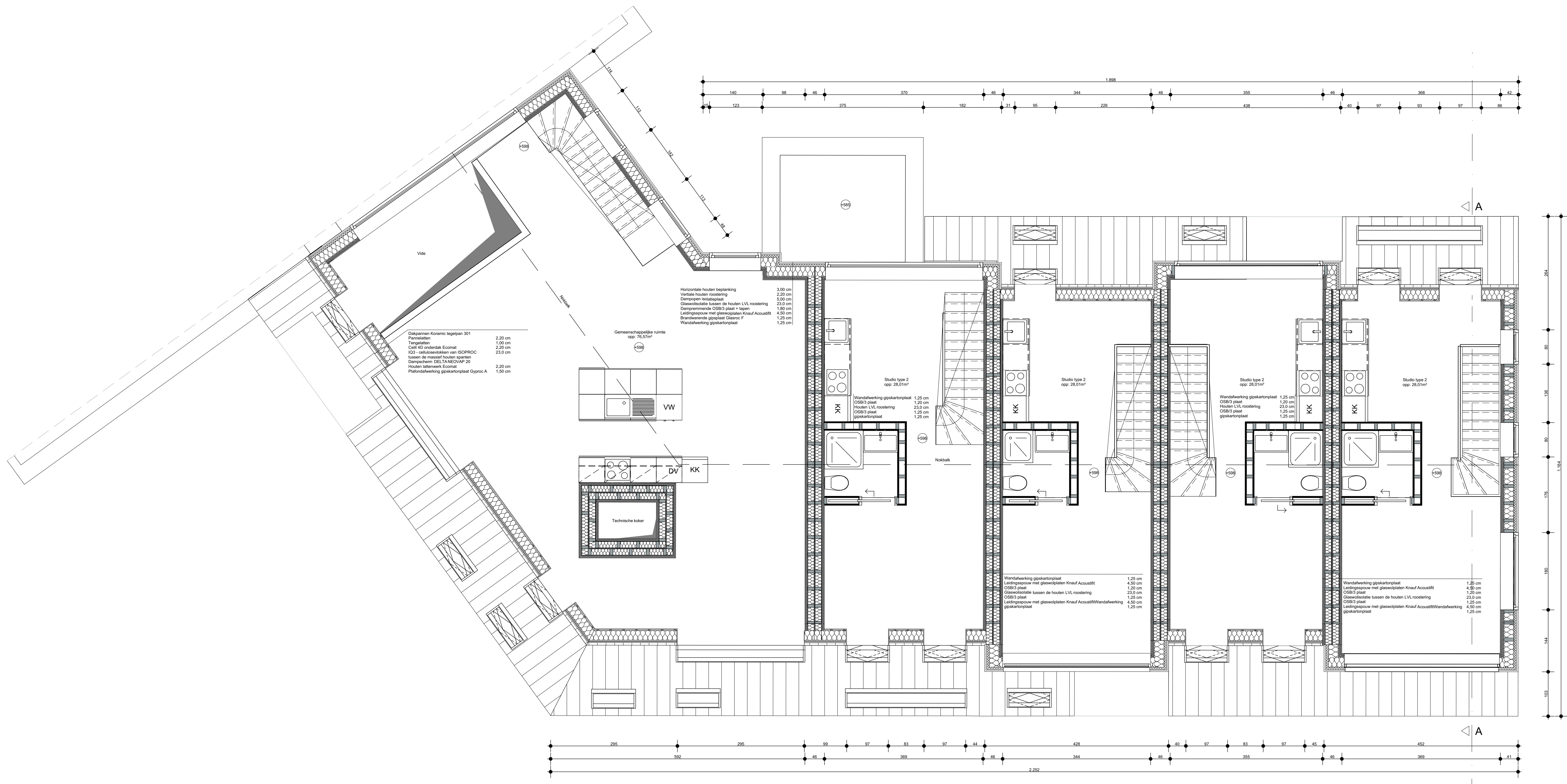
Grondplan tweede verdieping
